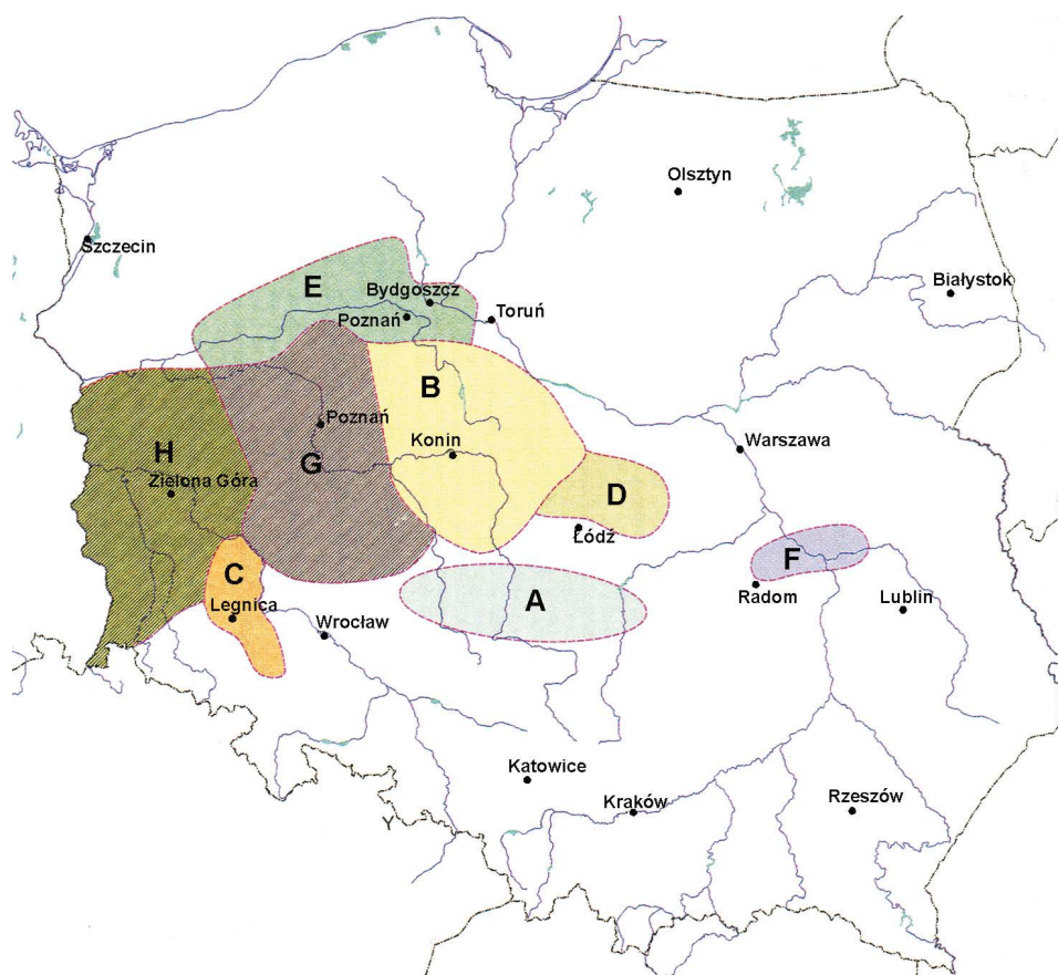
Rys. 2. Występowanie węgla brunatnego w Polsce z zaznaczeniem rejonów ich zalegania według Kasińskiego i in. (2016) A – rejon bełchatowski, B – rejon koniński, C – rejon legnicki, D – rejon łódzki, E – rejon północno-zachodni, F – rejon radomski, G – rejon wielkopolski, H – rejon zachodni
